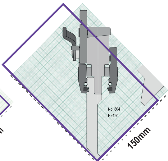
Nytt AFH (H=120mm) verktyg
